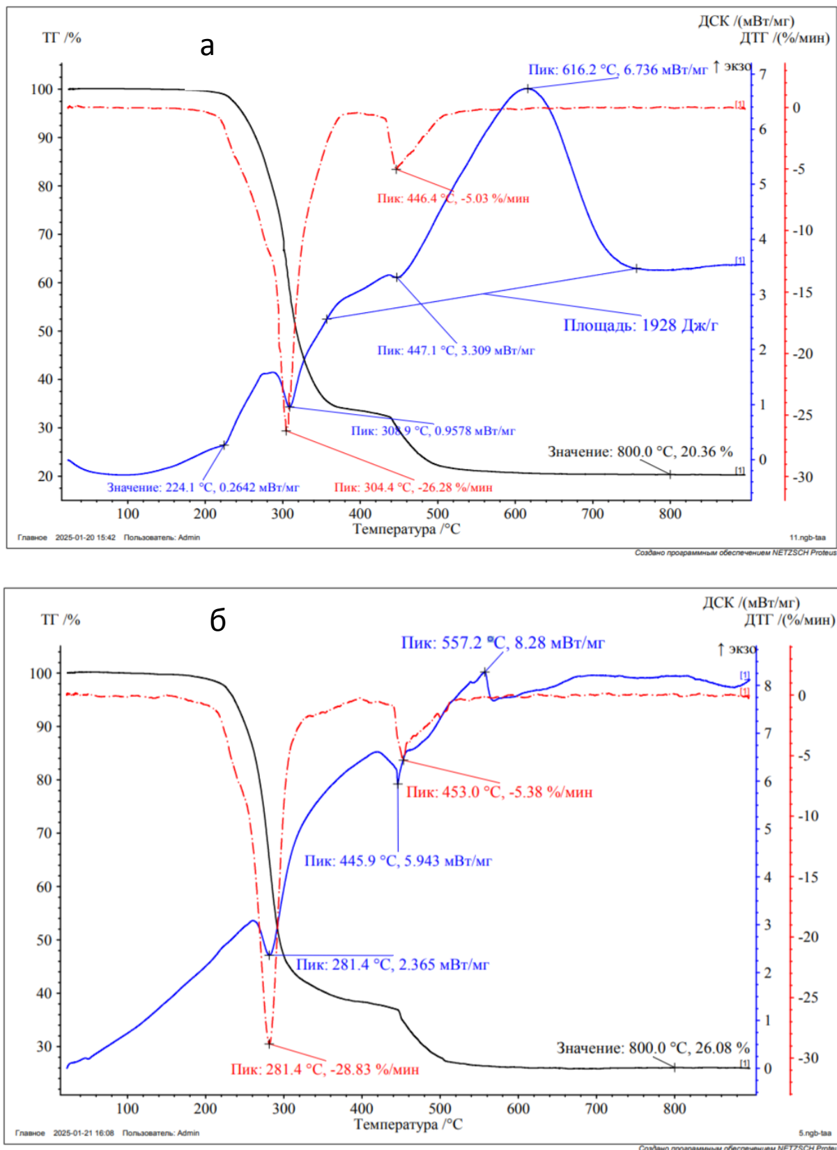
Рис. 1 Термограммы древесно-полимерного композита
