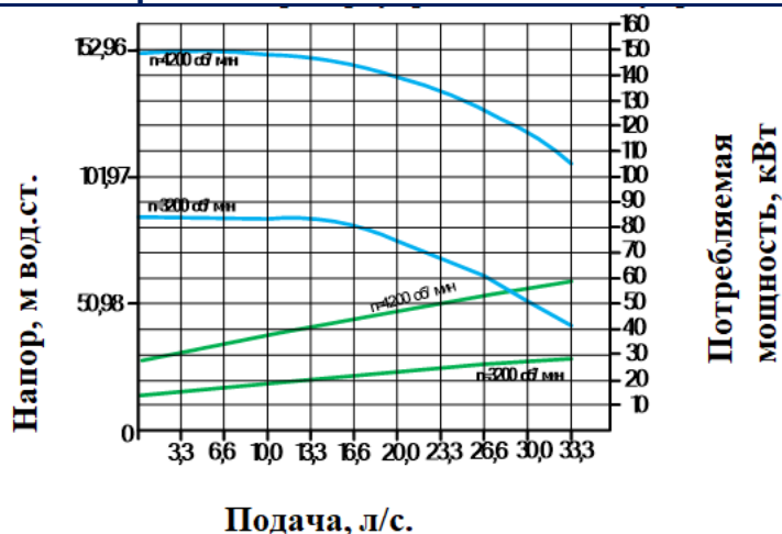
Рис.6. Напорно-энергетические характеристики насоса N20
