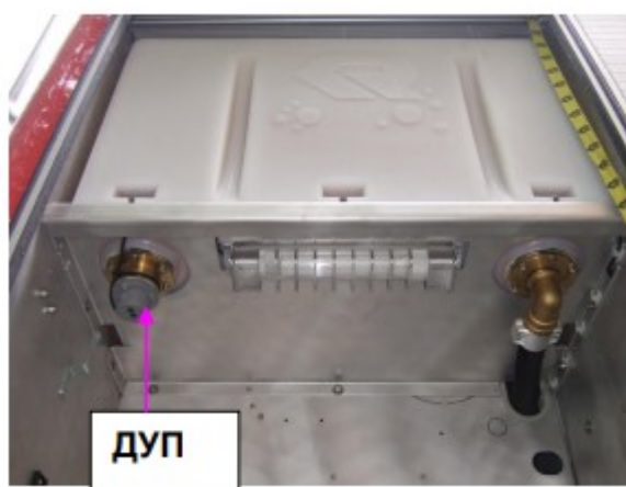
Рис.1 — Пенобак ПА АЦ-3,2-40-4(43253)001-МС
