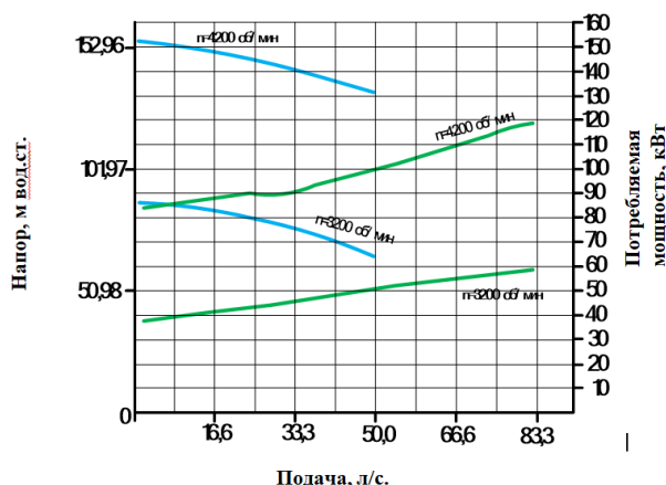
Рис.8. Напорно-энергетические характеристики насоса N30
