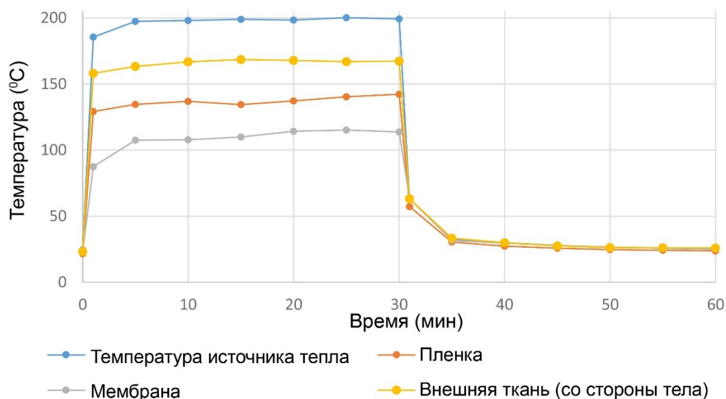
Рис. 2. Тепловые характеристики материалов, использованных в жилете, без интеграции АФП
