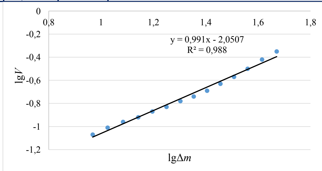
Рис. 2. Графическая зависимость логарифма скорости потери массы от логарифма потери массы ПЭВП
