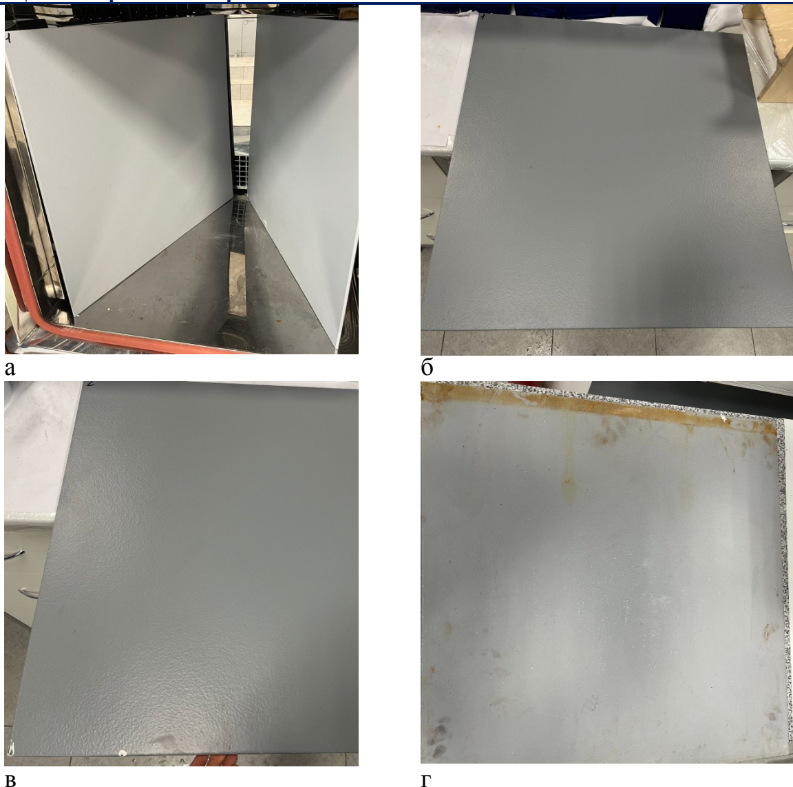
Рис. 1. Состояние покрытия: а – до климатических испытаний; б – после 45 циклов старения (5 лет); в – после 134 циклов старения (15 лет); г – после 224 циклов старения (25 лет)
